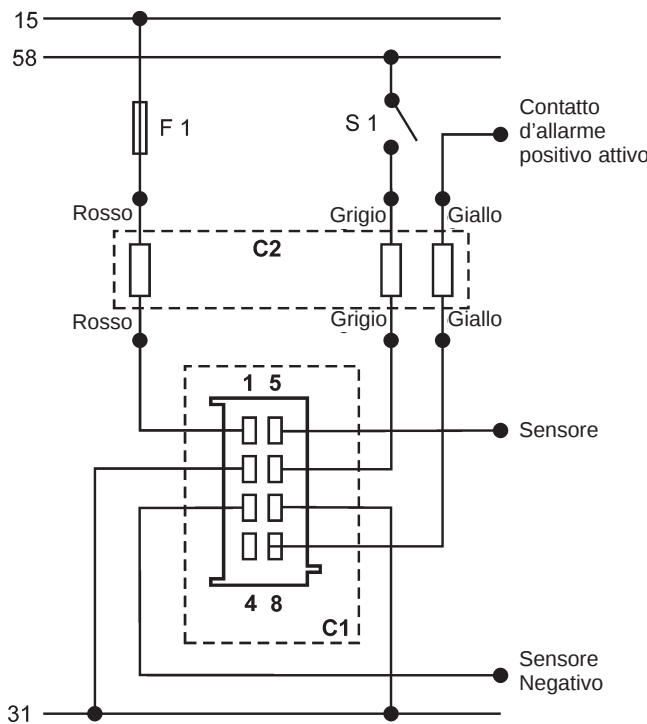
Variante 2: contatto d'allarme positivo attivo
